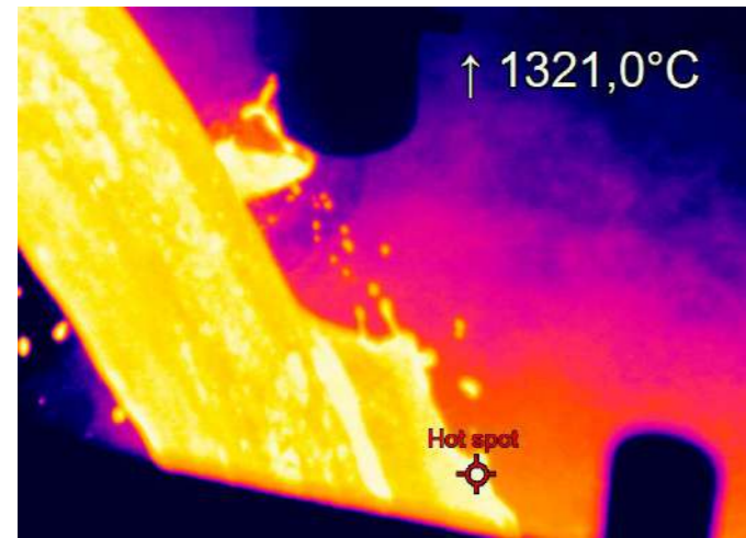
Gracias al rango de medición continuo de 900 a 2450 °C, el PI 05M es especialmente adecuado para la medición de temperatura de metales fundidos.
