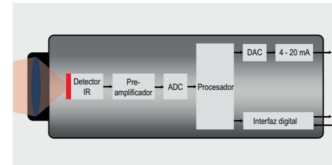
Esquema funcional de un termómetro de infrarrojo
